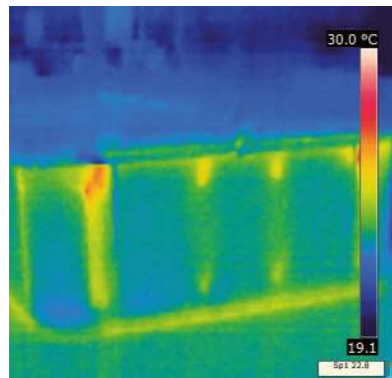
Test szczelności cieplnej przeprowadzony z izolacją Nordic
